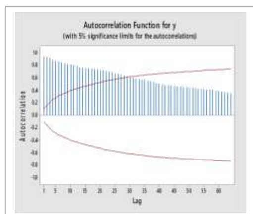
الشكل (2) : يمثل معامل الارتباط الذاتي لـ (y)
