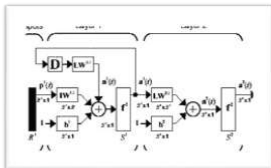
الشكل (1) : يوضح الشبكة العصبية المعادة RNN
