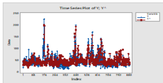
الشكل (8): التطابق بين البيانات الاصلية مع البيانات التقديرية (سلسلة التنبؤ) للمتغير المعتمد ( PM_{10} ) لبيانات التدريب باستخدام RNN-Wavelet الهجينة.
