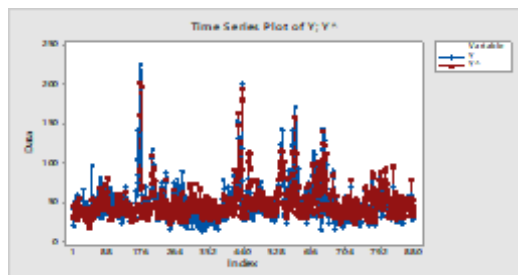
الشكل (6): التطابق بين البيانات الاصلية مع البيانات التقديرية (سلسلة التنبؤ) للمتغير المعتمد ( PM_{10} ) خلال الفترة الكلية لبيانات الاختبار باستخدام MLR-RNN. خلال الفترة الكلية لبيانات التدريب باستخدام MLR-RNN.
