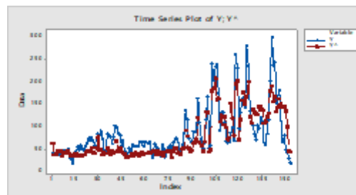
الشكل (6): التطابق بين البيانات الاصلية مع البيانات التقديرية (سلسلة التنبؤ) للمتغير المعتمد ( PM_{10} ) خلال الفترة الكلية لبيانات الاختبار باستخدام MLR-RNN. خلال الفترة الكلية لبيانات التدريب باستخدام MLR-RNN.
