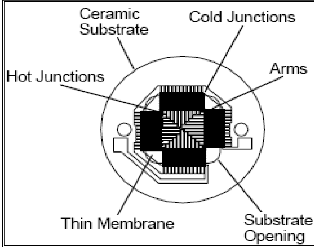
الشكل (١) مقطع عرضي يمثل أجزاء الثرموبايل
